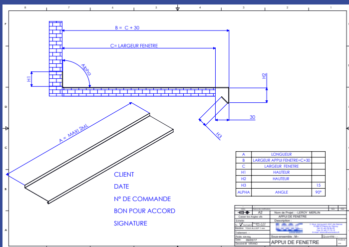
Exemple de plan pour un appui fenêtre
