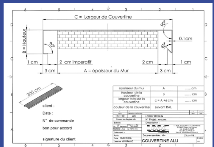
Exemple de plan pour une couvertine
