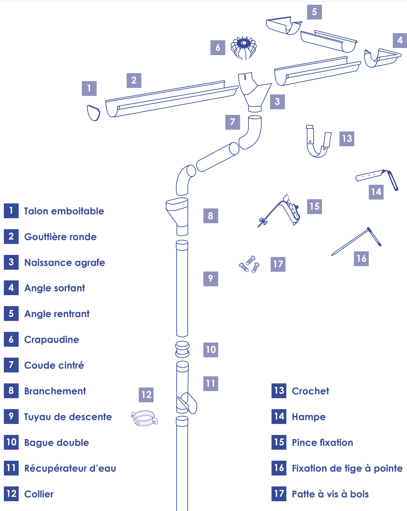
Schéma de montage d'une gouttière demi-ronde
